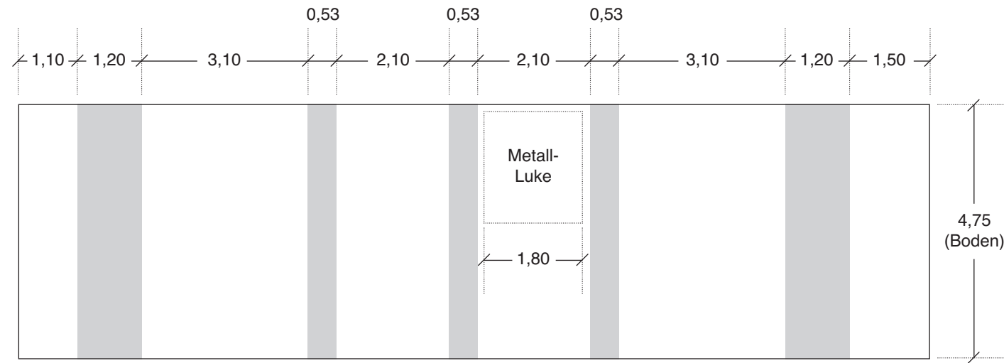
Draufsicht
